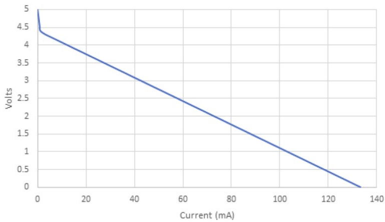
(d) Output voltage versus current output
